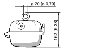
Tornillo de cáncamo montado en tuerca autoinsertable de la luminaria
