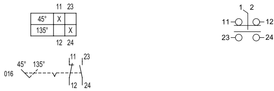
Esquema de conmutación 8008/-016
