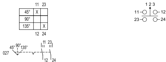
Esquema de conmutación 8008/-.027
