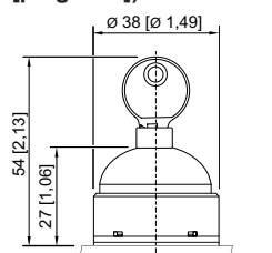
Interruptor de llave 8003/...-008
