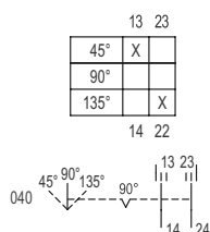
Esquema de conmutación 8008/-040
