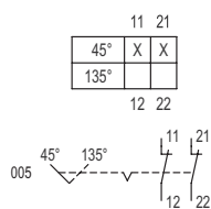
Esquema de conmutación 8008/-005
