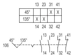
Esquema de conmutación 8008/2-106 Esquema de conmutación 8008/4-11-06
