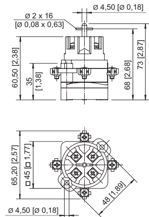
8008/2-1 combinador de control 3 o 4 polos
