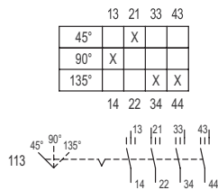
Esquema de conmutación 8008/2-113 Esquema de conmutación 8008/4-11-13
