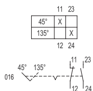
Esquema de conmutación 8008/-016
