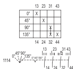
Esquema de conmutación 8008/-1114
