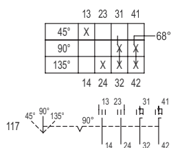
Esquema de conmutación 8008/-117
