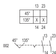
Esquema de conmutación 8008/-002
