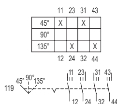
Esquema de conmutación 8008/-119
