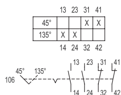
Esquema de conmutación 8008/.-106
