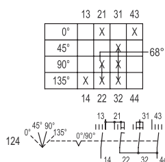
Esquema de conmutación 8008/-124
