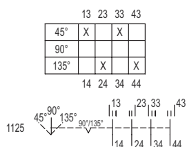
Esquema de conmutación 8008/-1125
