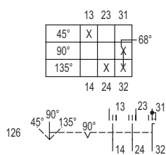
Esquema de conmutación 8008/-126
