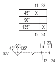
Esquema de conmutación 8008/2-027 Esquema de conmutación 8008/4-10-27
