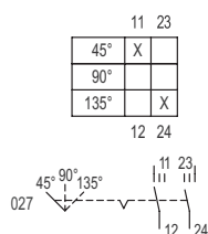
Esquema de conmutación 8008/-027
