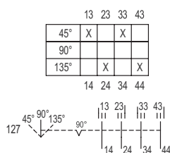
Esquema de conmutación 8008/.-127
