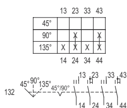
Esquema de conmutación 8008/-132
