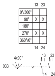
Esquema de conmutación 8008/2-033 Esquema de conmutación 8008/4-10-33
