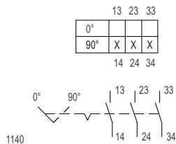
Esquema de conmutación 8008/2-1140 Esquema de conmutación 8008/4-11-140
