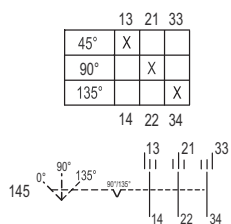
Esquema de conmutación 8008/.-145
