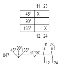
Esquema de conmutación 8008/2-047 Esquema de conmutación 8008/4-10-47
