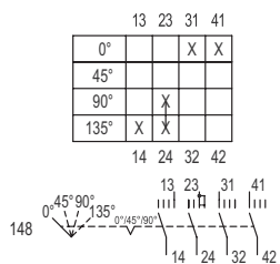
Esquema de conmutación 8008/-148
