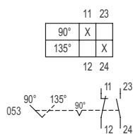
Esquema de conmutación 8008/-053
