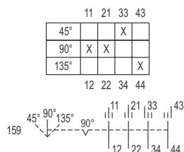
Esquema de conmutación 8008/-159
