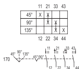
Esquema de conmutación 8008/.-170
