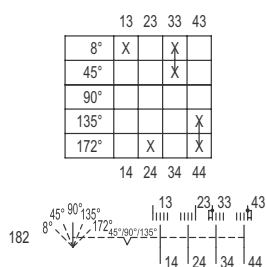
Esquema de conmutación 8008/-182
