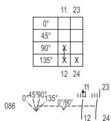
Esquema de conmutación 8008/-086
