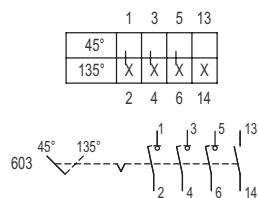
Esquema de conmutación 8008/-603
