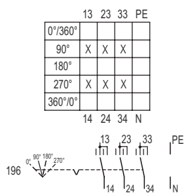
Esquema de conmutación 8008/-196
