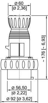
Enchufe de 5 polos
