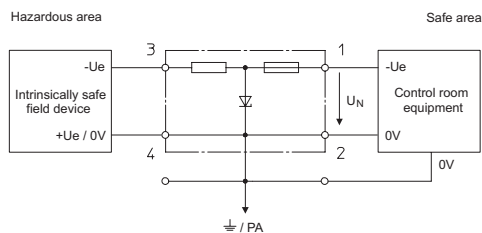
Barreras de seguridad intrínseca de un canal para potencial negativo
