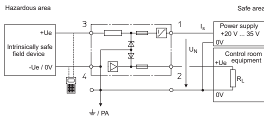
Barreras de seguridad intrínseca de un canal para transductores
