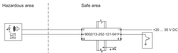
Caso de aplicación: salida analógica (fuente de corriente) para convertidor i/p etc. Circuito de campo conectado flotante
