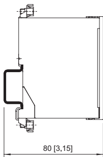
Montado en riel de montaje DIN NS 35/15
