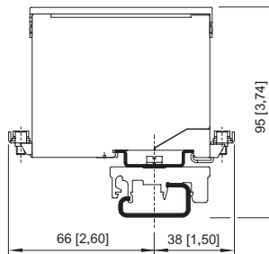
Montado en riel de montaje DIN NS 32 con adaptador y pie de sujeción de plástico moldeado
