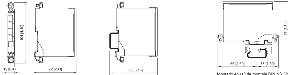
Montado en raíl de montaje DIN NS 35/15
