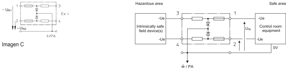
Barreras de seguridad intrínseca de dos canales para potencial -/-
