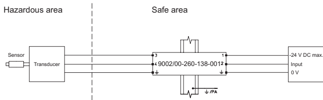
Caso de aplicación: sensor de vibraciones
