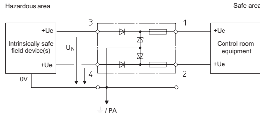
Barreras de seguridad intrínseca de dos canales Potencial de barrera de evaluación: + / Potencial de barrera de evaluación: +
