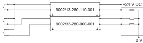
Caso de aplicación: combinación de contactos sin potencial
