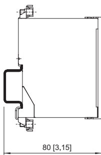
Montado en raíl de montaje DIN NS 35/15
