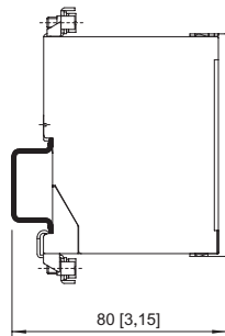
Montado en carril de montaje DIN NS 35/15
