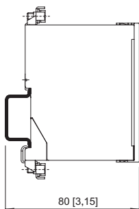
Montado en carril de montaje DIN NS 35/15
