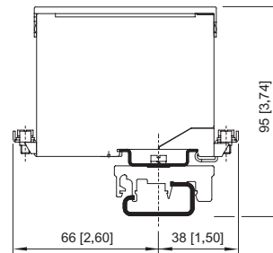
Montado en carril de montaje DIN NS 32 con adaptador y pie de sujeción de plástico moldeado
