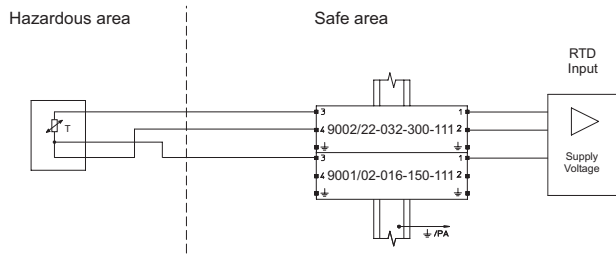
Caso de aplicación: Pt100, circuito de campo flotante de conexión de 3 conductores
