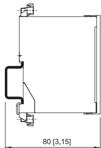
Montado en raíl de montaje DIN NS 35/15
