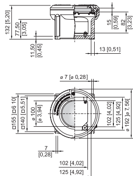
Tamaño de carcasa 2 con mirilla
