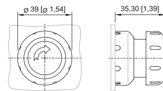
8602/3-010 Pulsador de seta enclavable rojo/amarillo 8602/3-012 Pulsador de seta enclavable negro/negro Actuador con accionamiento axial
