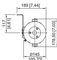
Señal acústica GRP, serie YA6S con estribo en L
