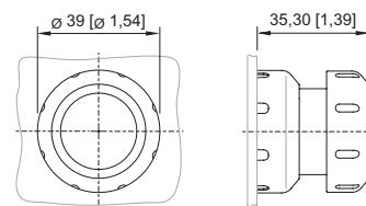
8602/3-003 Pulsador seta negro 8602/3-004 Pulsador seta rojo/negro Actuador con accionamiento axial
